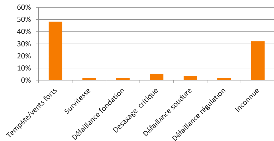
Figure 8 : Répartition des causes premières d'effondrement dans les accidents à l'international entre 2000 et 2011
