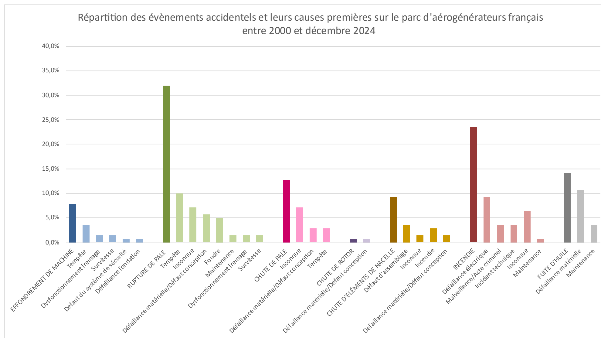
Figure 6 : Répartition des accidents et de leurs causes premières sur le parc éolien français entre 2000 et décembre 2024 (Source : ENCIS Environnement, d'après le Guide technique, mai 2012)
